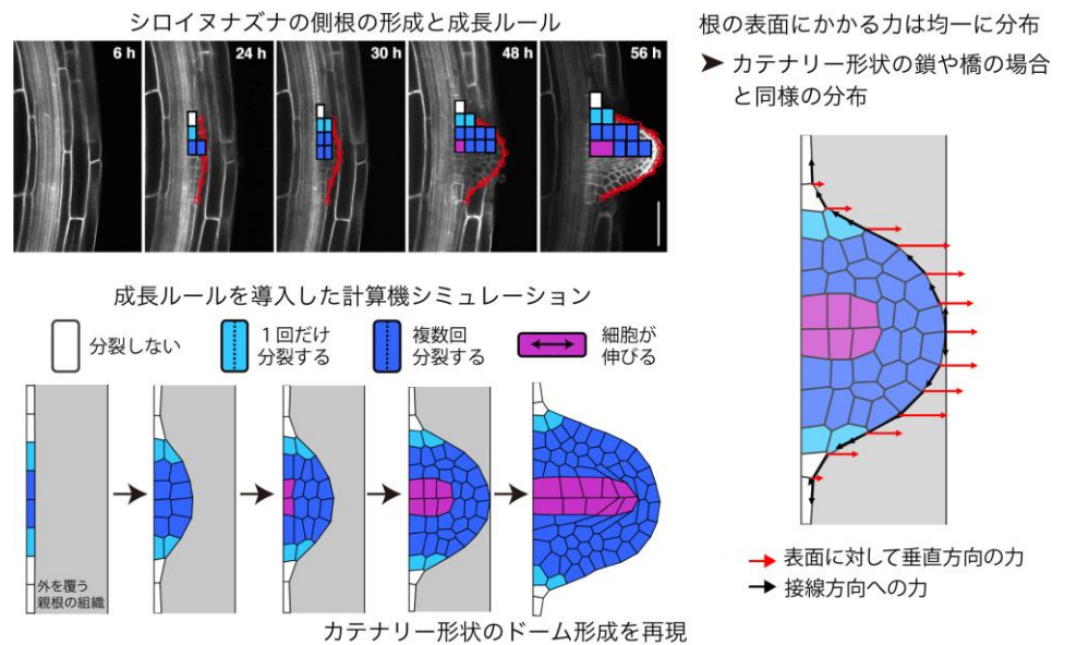
図3 カテナリー曲線の成り立ち。シロイヌナズナの側根の発生過程(左上)の細胞分裂の性質を導入した計算機シミュレーション(左下)を行い、根の表面にかかる力を計算(右)。
