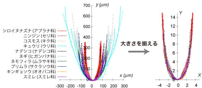
図2 根の輪郭の形は種を超えて共通する。 10種の主根の輪郭(左)を、カタナリー曲線の曲率半径 a で割る(右)。
